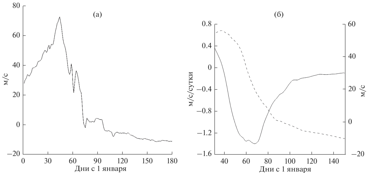
Рис. 1. Изменение среднезонального ветра (м/с) (а), сглаженное изменение среднезонального ветра (м/с) (пунктирная линия, правая шкала) и сглаженная скорость его изменения (м/с/день) (сплошная линия, левая шкала) (б) на 10 гПа и 62.5° с.ш. с 1 февраля по 31 мая 1987 г. по данным реанализа ERA-Interim.
